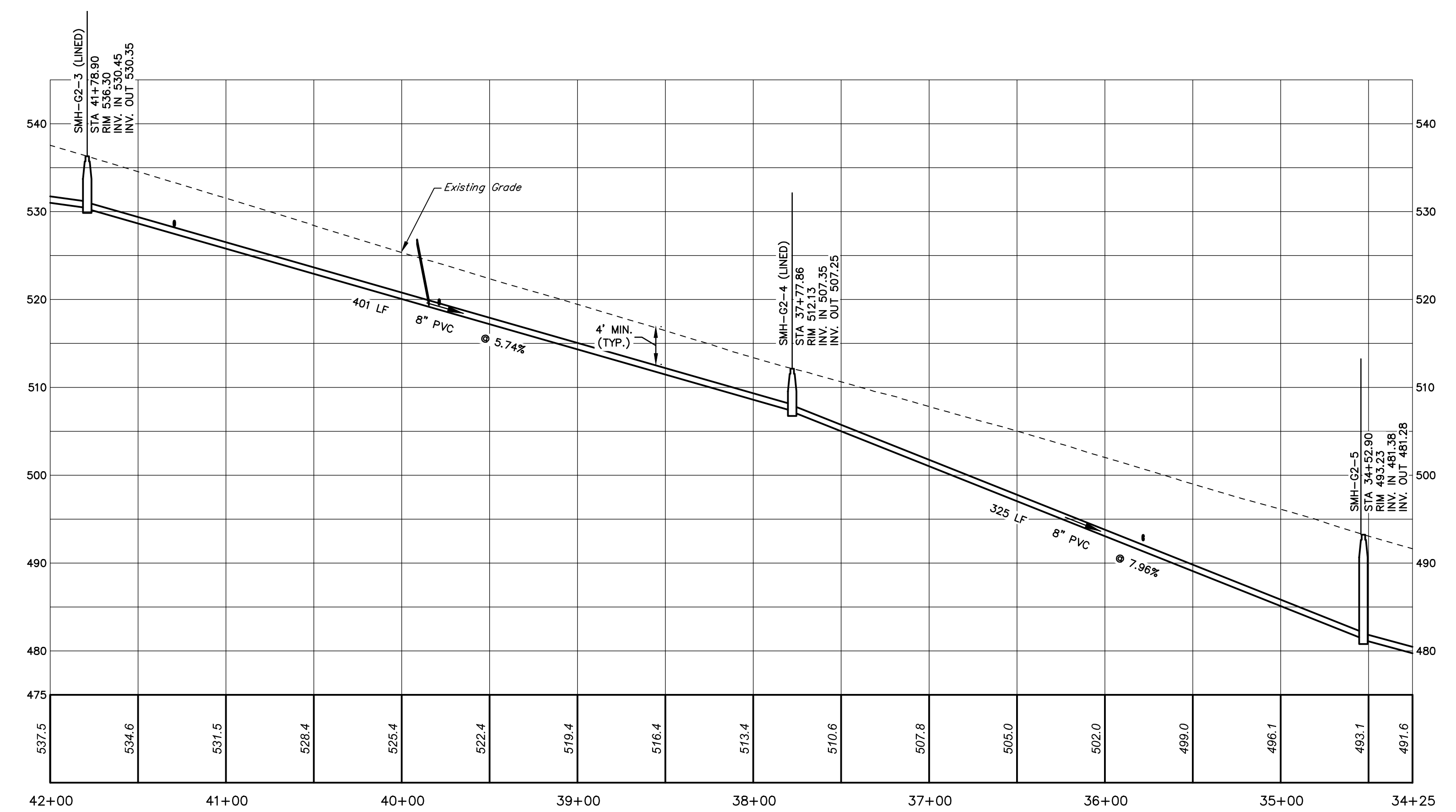
PROFILE HORIZ. SCALE: 1" = 50' VERT. SCALE: 1" = 10'
