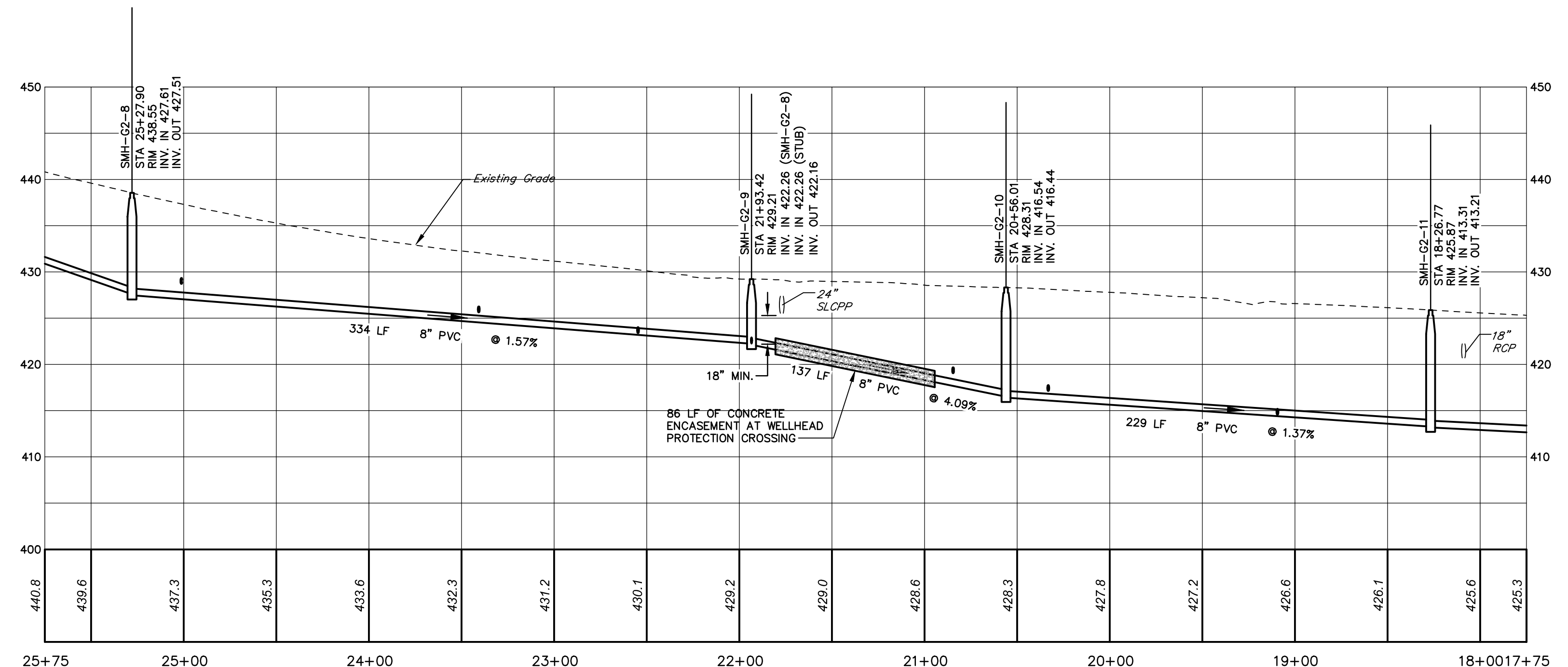
PROFILE HORIZ. SCALE: 1" = 50' VERT. SCALE: 1" = 10'
