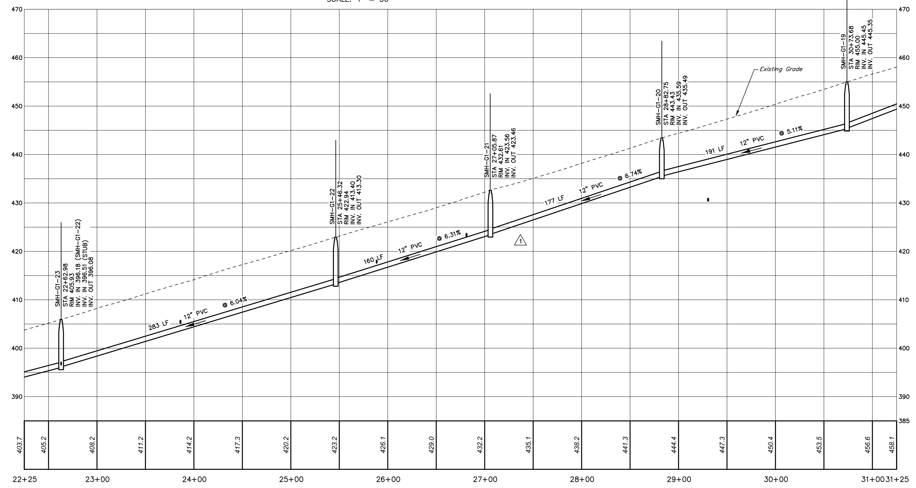
PROFILE HORIZ. SCALE: 1" = 50' VERT. SCALE: 1" = 10'
