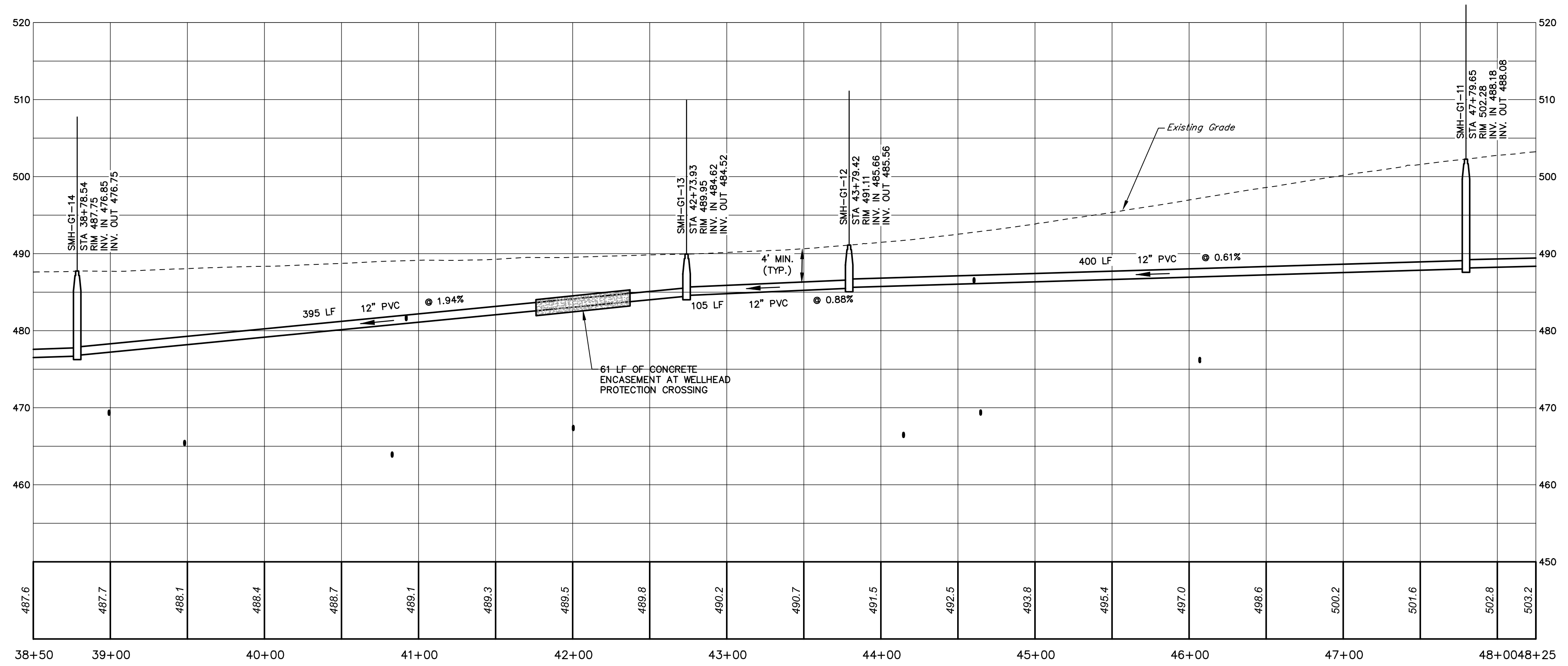
PROFILE HORIZ. SCALE: 1" = 50' VERT. SCALE: 1" = 10'
