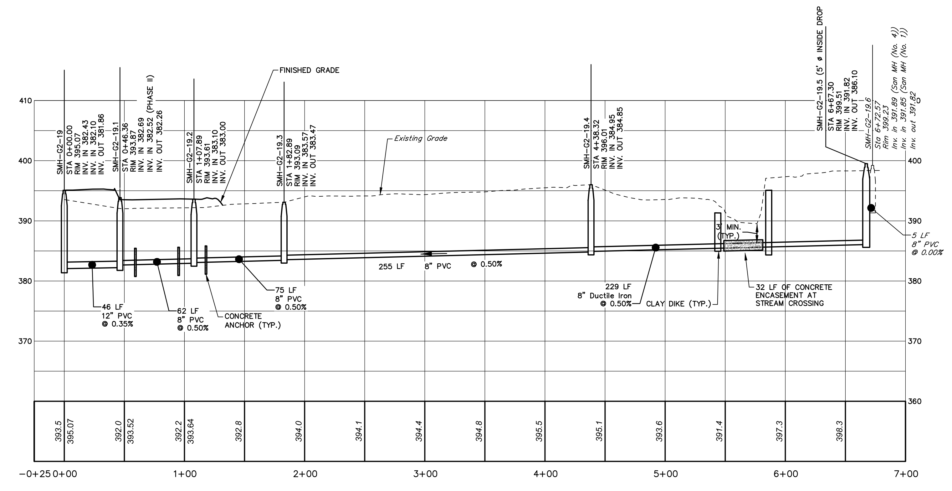
PROFILE HORIZ. SCALE: 1" = 50' VERT. SCALE: 1" = 10'
