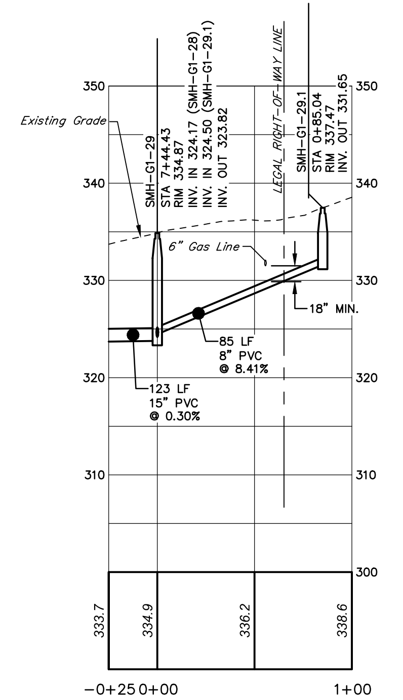
PROFILE HORIZ. SCALE: 1" = 50' VERT. SCALE: 1" = 10'
