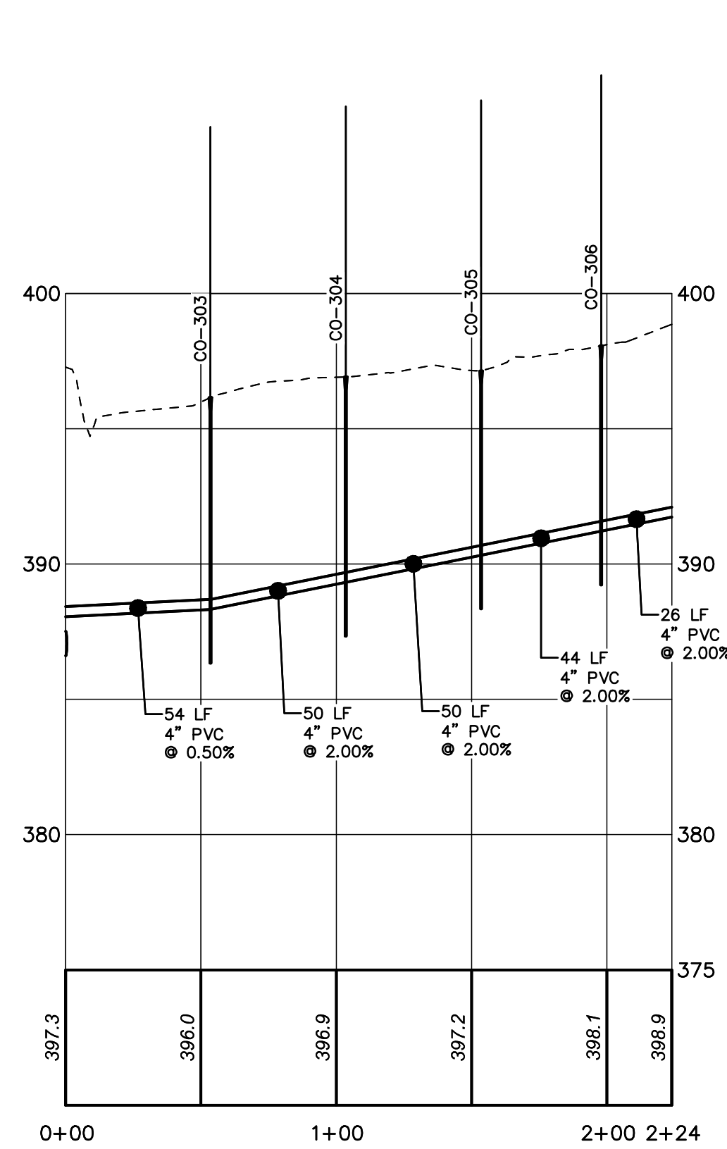
PROFILE HORIZ. SCALE: 1"=50' VERT. SCALE: 1"=5'
