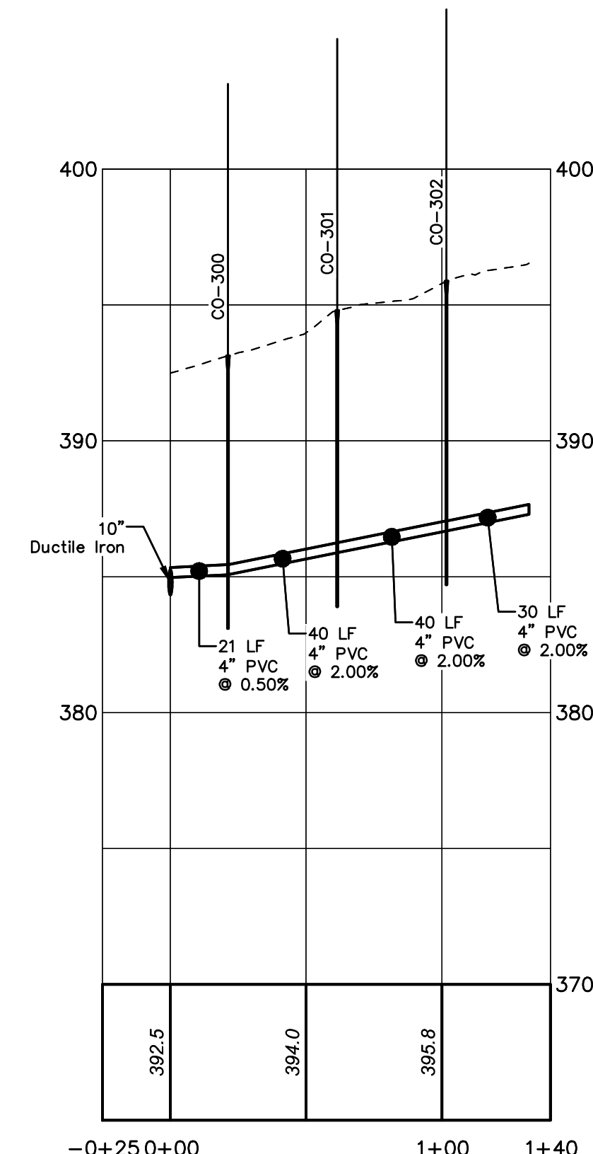
PROFILE HORIZ. SCALE: 1"=50' VERT. SCALE: 1"=5'
