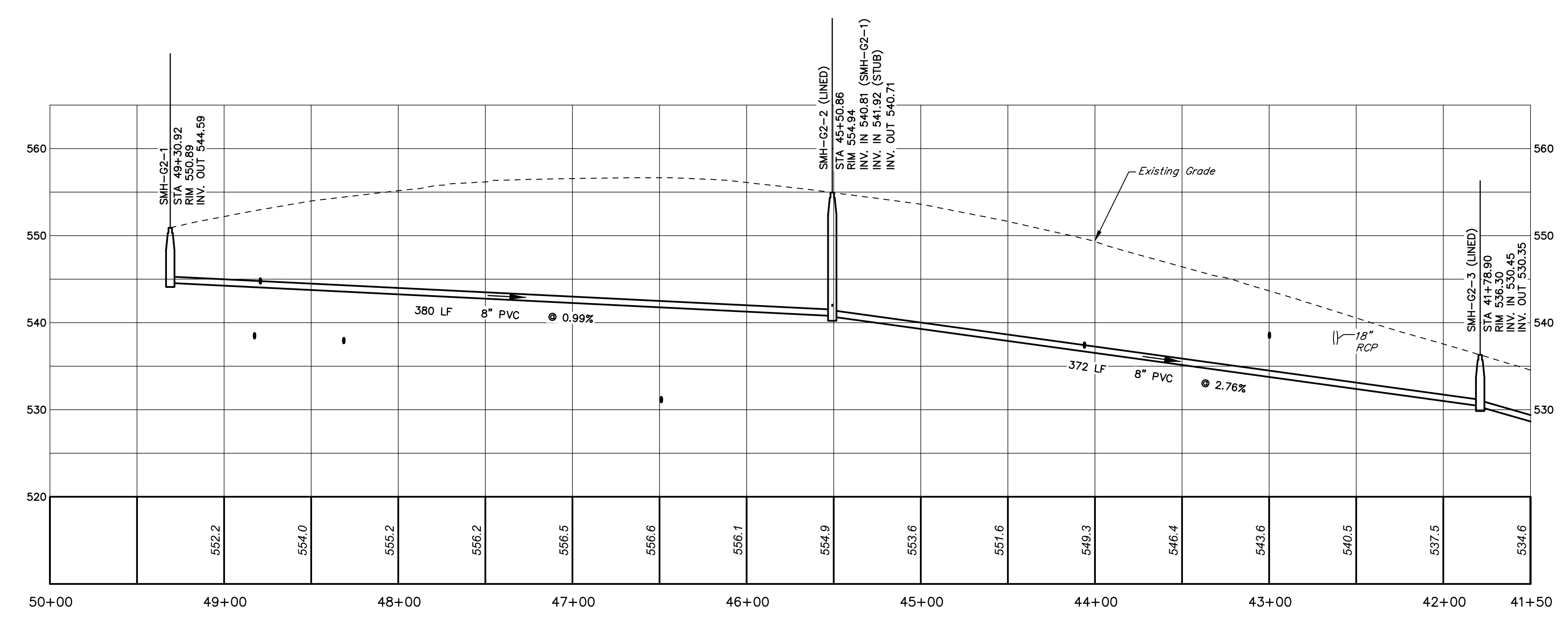
PROFILE HORIZ. SCALE: 1" = 50' VERT. SCALE: 1" = 10'
